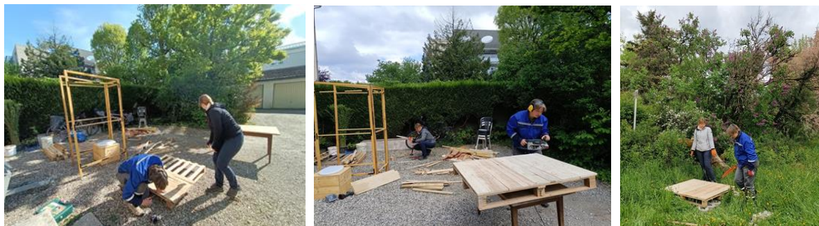
Photos du chantier de construction de la cabine de toilette sèches
